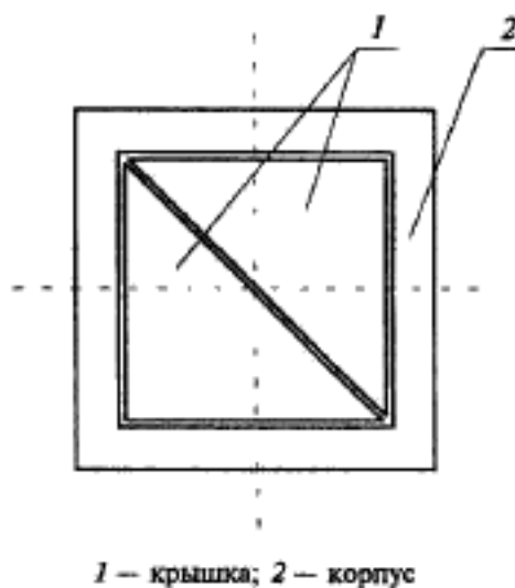
Рисунок А.5 — Люк с крышкой, состоящей из двух частей
