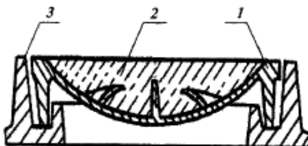
Рисунок А.2 — Люк, оснащенный запорным замковым устройством
